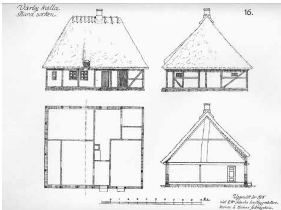
Uppmåtningsritning utförd 1916 vid landbyggmästarekursen, Hvilans folkhögskola.
