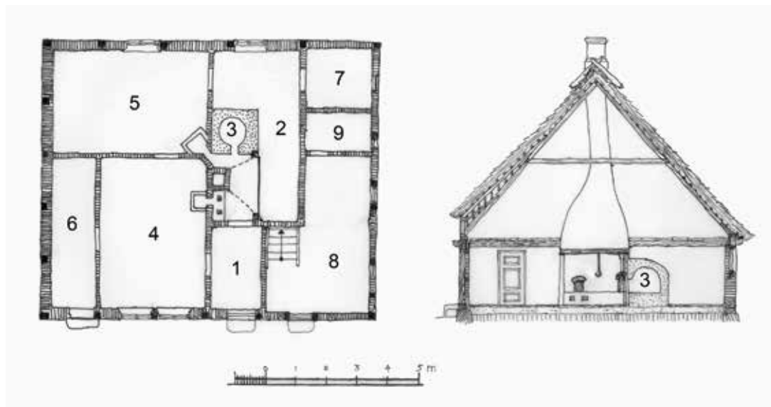
Rekonstruktionsförslag av Killehusets ursprungliga planlösning. 1: Förstuga. 2: Kök med ”illare”. 3: Bakugn. 4: Sal med sättugn. 5: Kammare med ugn. 6: Kistekammare. 7: Spiskammare. 8: Förråd med trapp till loftet. 9: Vedförråd. Kökets utformning är hypotetisk men kan ha varit utformad som på rekonstruktionen.
