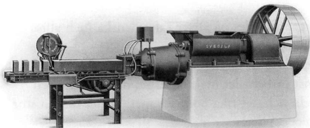
En murtegelpress av typ som tillverkades hos Åbjörn Anderssons Mekaniska verkstad.
