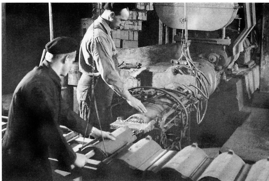
Elever fick också deltaga i praktiskt arbete. Här vid en Tegelpress för taktegel.
