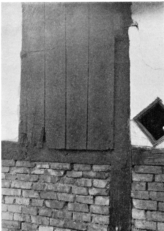
Vägg med lämm och glugg intill loggolvet. Nedanför löshultet lerkliningens ersatt med tegel.
