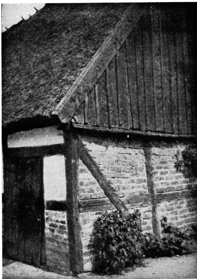
Klinevägg ersatt med tegel med bibehållande av korsvirket. Knästorp n:r 4. Hörn av loglänga, uppförd 1810.
